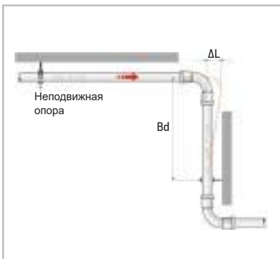
Рис. 46. Z-образный компенсатор.
